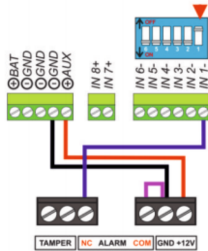
روش نصب سنسور باسیم
