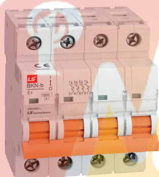
BKN-b 3P+N
