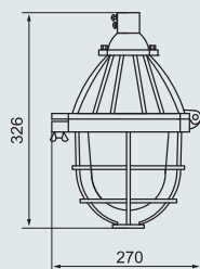
HRD51-150
