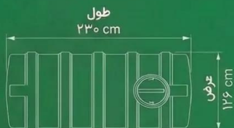
نمای بالا
