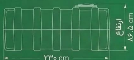
نمای جلو
